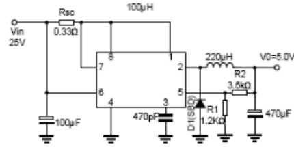
图2 降压变换器
