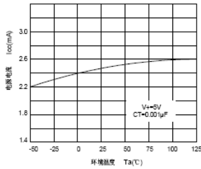
电源电流与温度关系
