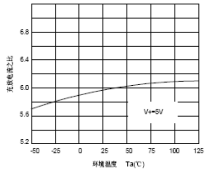
充放电电流之比与温度关系
