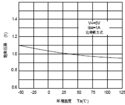
饱和压降 (1)与温度关系
