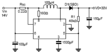
图1 升压变换器
