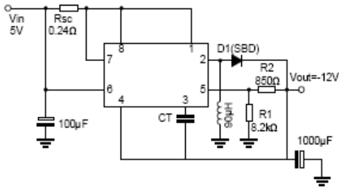
图5 反向变换器
