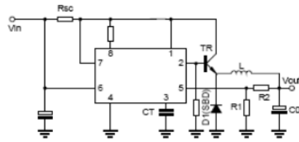
图4 降压变换器(大电流)
