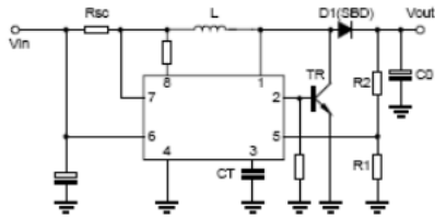
图3 升压变换器 (大电流)
