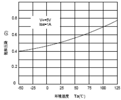
饱和压降 (2)与温度关系
